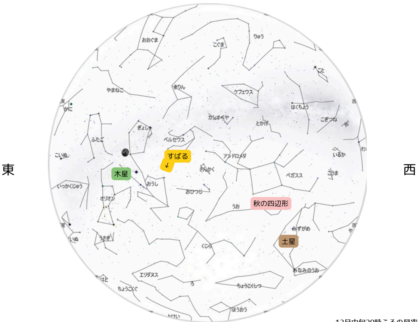
12月中旬20時ごろの星空 Stella Navigator12にて作成
